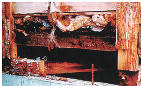
壁内に結露が発生し木材が腐朽した事例
